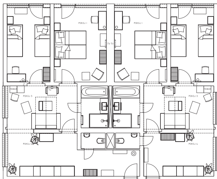
Půdorys nového řešení apartmánů DE LUXE a vizualizace provedení CLASSIC (foto nahoře vlevo) a MODERN (vpravo).
